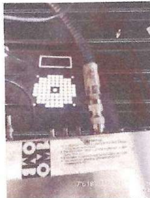
Figura-5 Instalación y reemplazo de transición N-N en TX - Radioenlace MW
