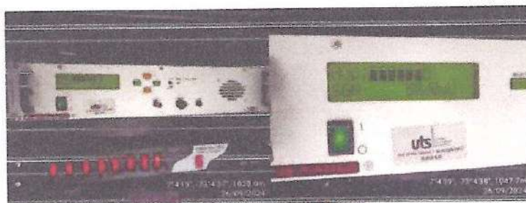
Figura-9 Instalación RX - Radioenlace MW
